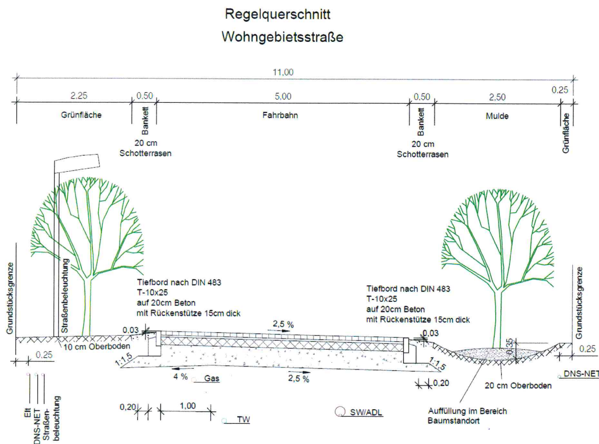
Abbildung 7: Straßenquerschnitt mit Versickerung
